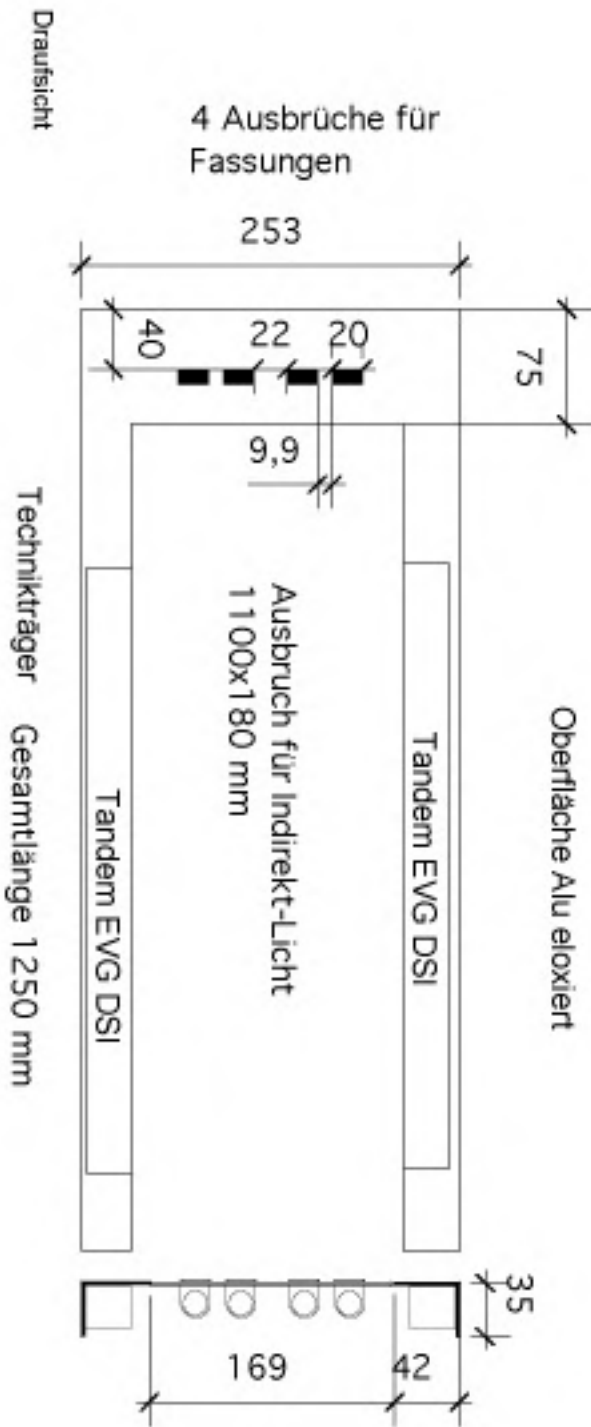
Schnitt Technikwanne
