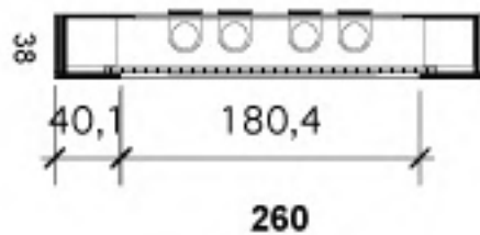
Schnitt Leuchtenwanne
